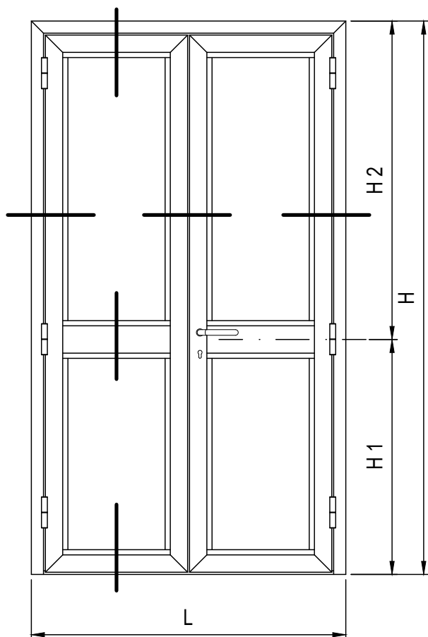
PROSPETTO INTERNO
