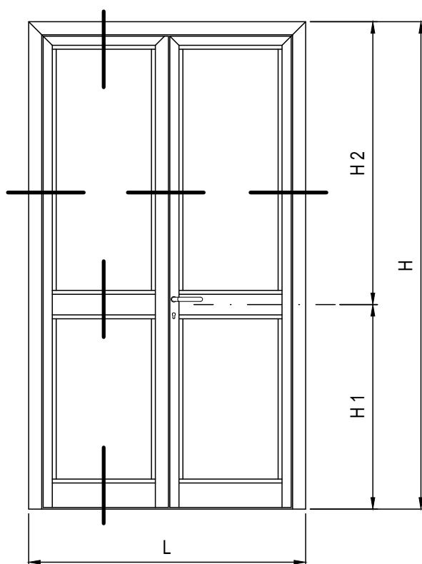
PROSPETTO INTERNO
