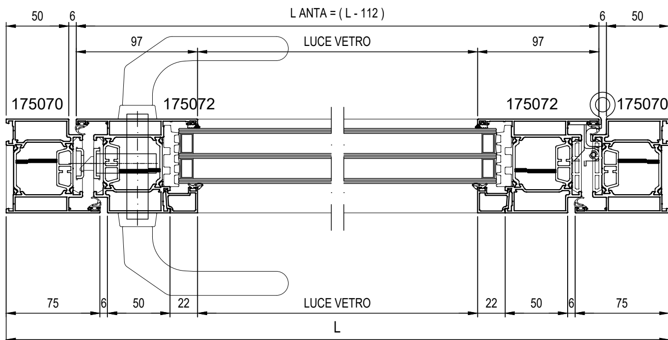
PROSPETTO INTERNO
