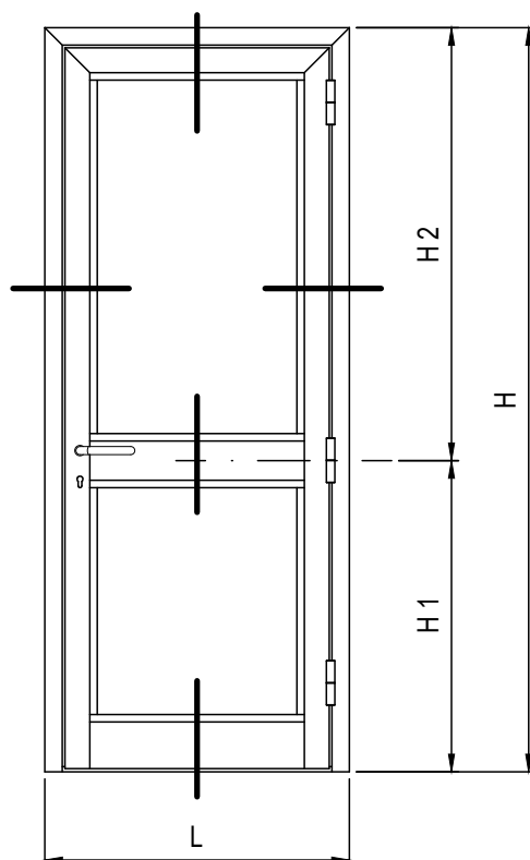
PROSPETTO INTERNO
