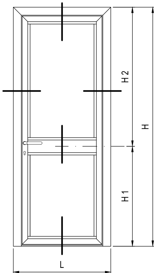
PROSPETTO INTERNO
